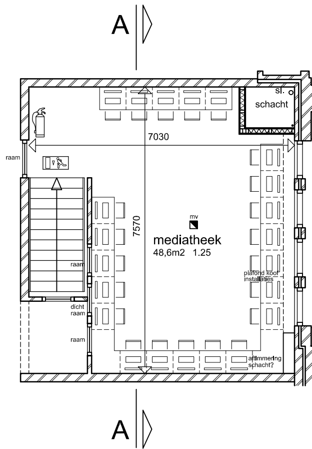
plattegrond tussenverdieping
